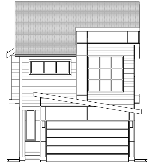
ELEVATION 2
